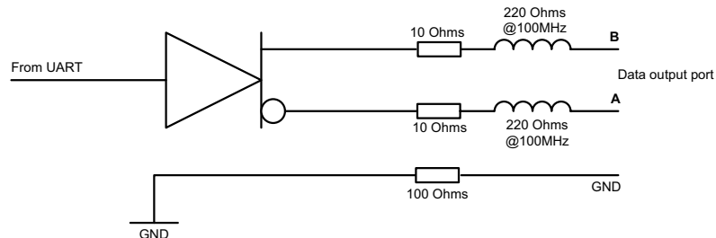
Afbeelding 55 Schema gegevensuitvoerpoort
