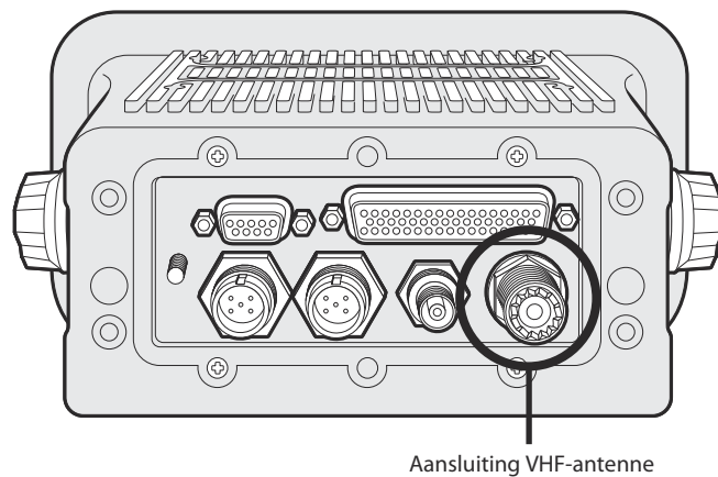
Afbeelding 42 Aansluiting VHF-antenne
