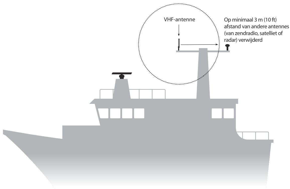
Afbeelding 41 Installatie van VHF-antenne
