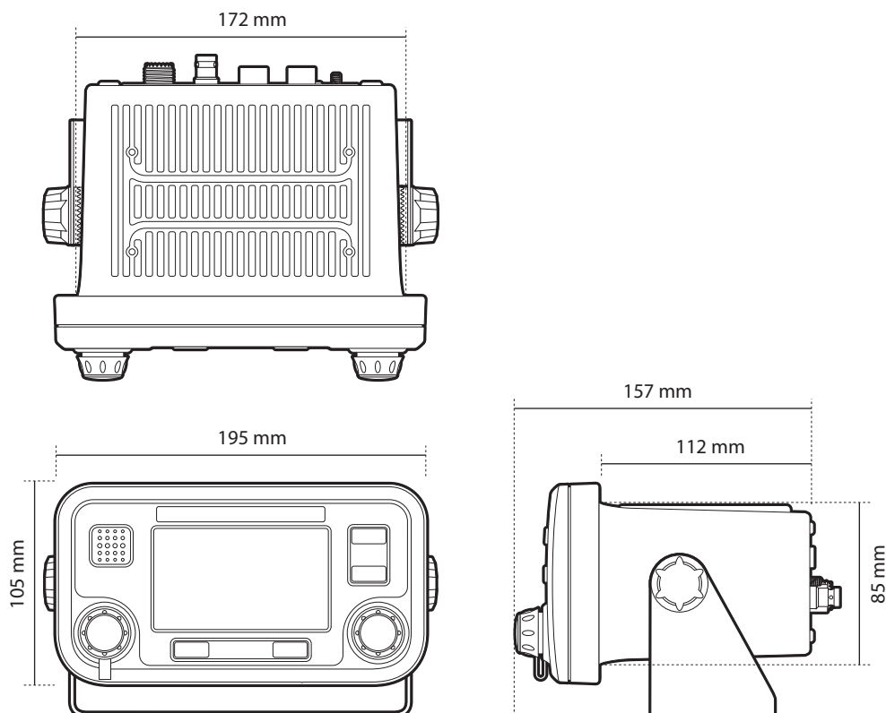
Afbeelding 34 Afmetingen van AIS-transponder
