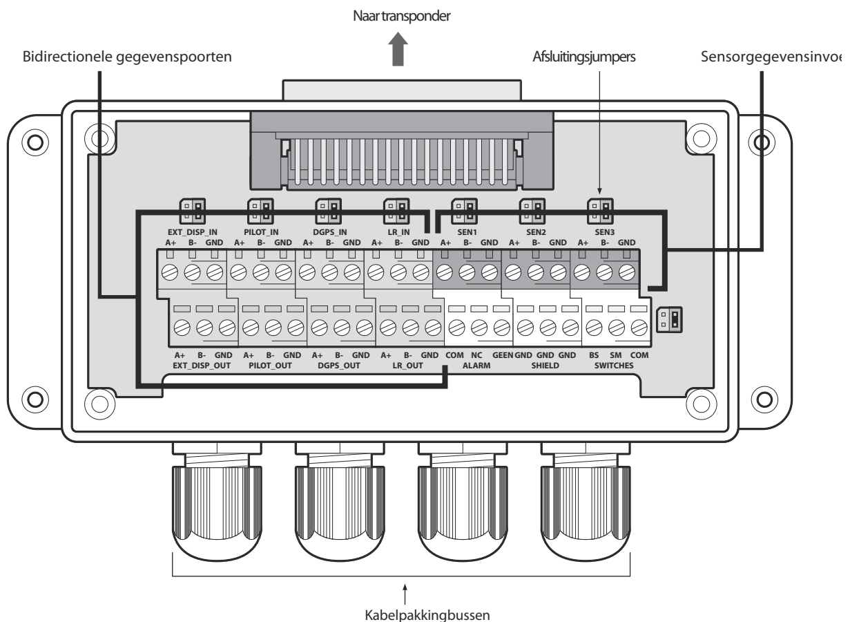
Afbeelding 44 Aansluitingen aansluitkast
