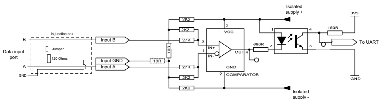
Afbeelding 54 Schema ingangspoort
